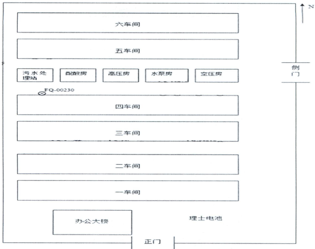
图1 厂区平面布置及监测点位分布图
